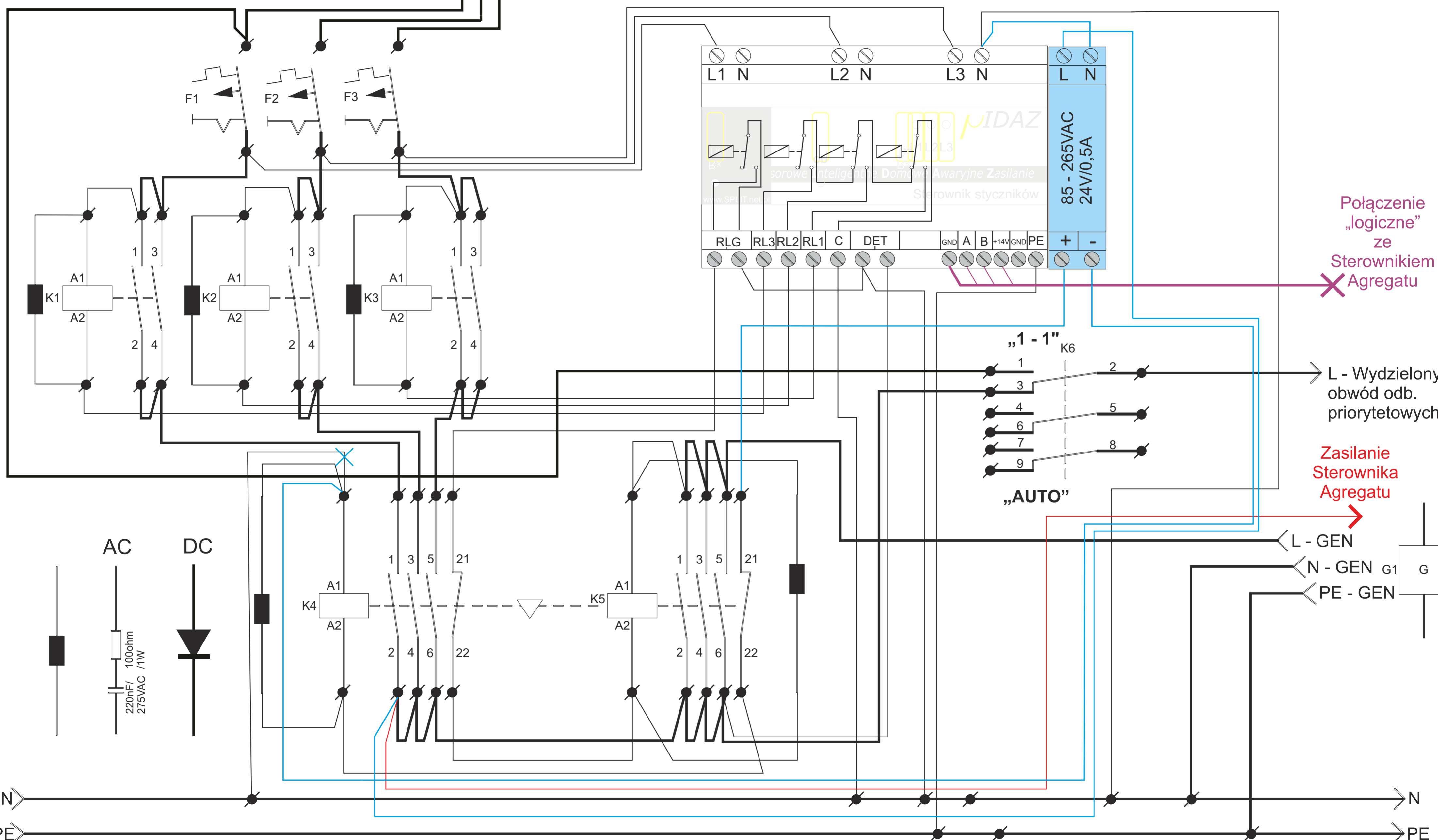
SCHEMAT PODŁĄCZENIA STYCZNIKÓW ZE STEROWNIKIEM W DODATKOWEJ ROZDZIELNICY SZR W INSTALACJI Z AGREGATEM JEDNOFAZOWYM (1F) Z WYDZIELONYM OBWODEM (JEDNOFAZOWYM) ODBIORNIKÓW „PRIORYTETOWYCH”
